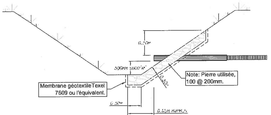
Coupe transversale
