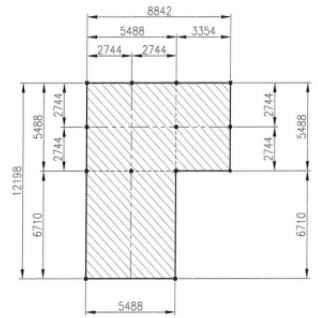
POSITIONNEMENT DES SONOTUBES
